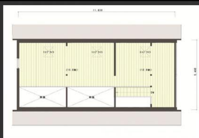
【 2F モデル FLOOR PLAN 】
